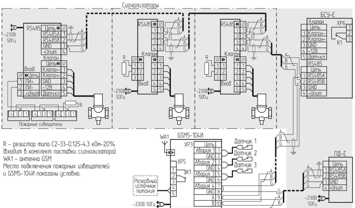
Рисунок Б.2 – Схема соединений системы с RS485 и индивидуальной защитой.
