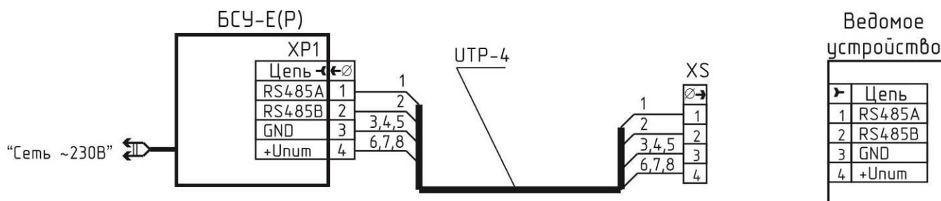
Рисунок К.1 – Схема соединений для программирования адресов
