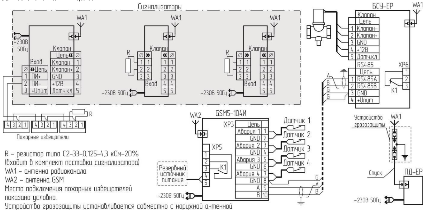
Рисунок Б.3 – Схема соединений системы с радиоканалом и групповой защитой.
