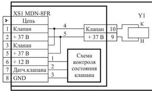
а) с разъемом MDN-8FR
