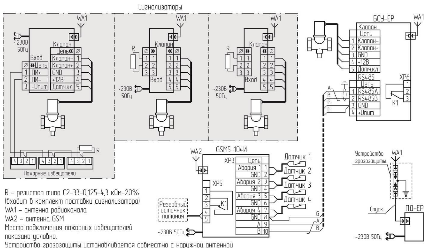
Рисунок Б.4 – Схема соединений системы с радиоканалом и индивидуальной защитой.
