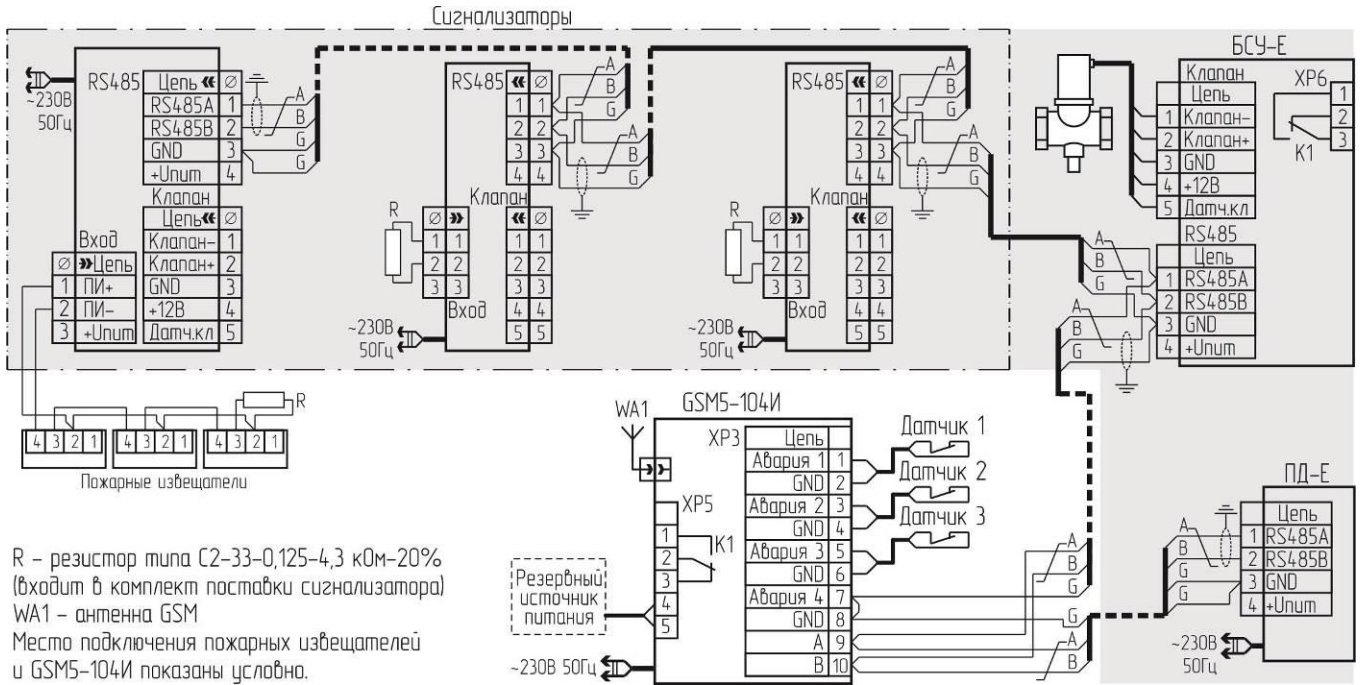
Рисунок Б.1 – Схема соединений системы с RS485 и групповой защитой.
